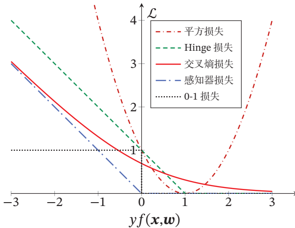
图 3.7 不同损失函数的对比
