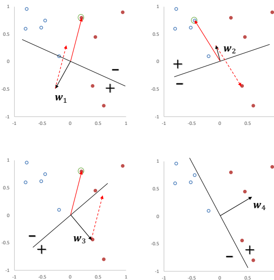
图 3.5 感知器参数学习的更新过程
