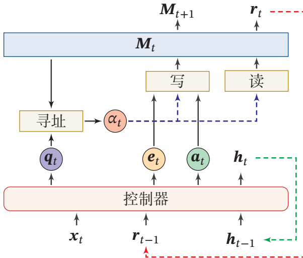
图 8.9 神经图灵机示例
