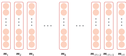
图 15.2 嵌入矩阵
