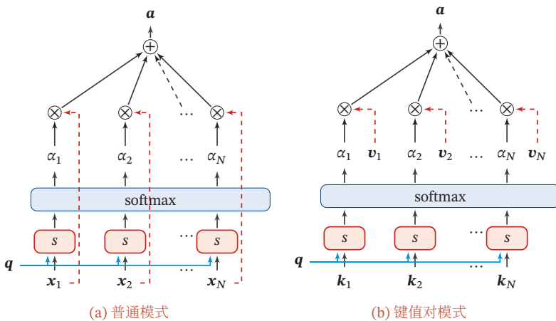
图 8.1 注意力机制
