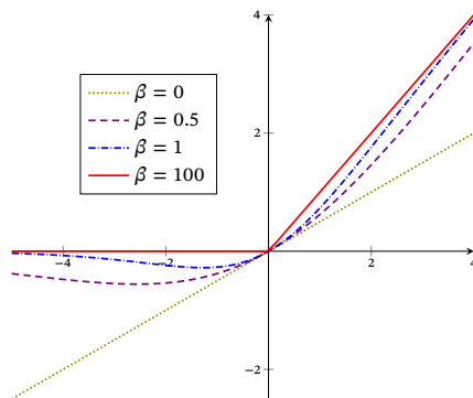
图 4.5 Swish 函数
