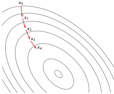
图 C.1 梯度下降法
