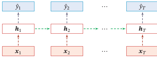
图 7.14 变分丢弃法
