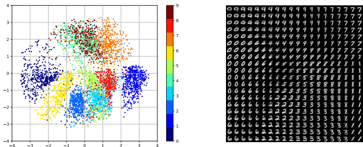
(a) 训练集上所有样本在隐空间上的投影 (b) 隐变量 \mathbf{z} 在图像空间的投影
