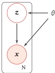
图 11.10 带隐变量的贝叶斯网络
