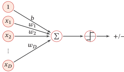
图 3.1 二分类的线性模型
