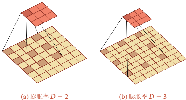
图 5.18 空洞卷积
