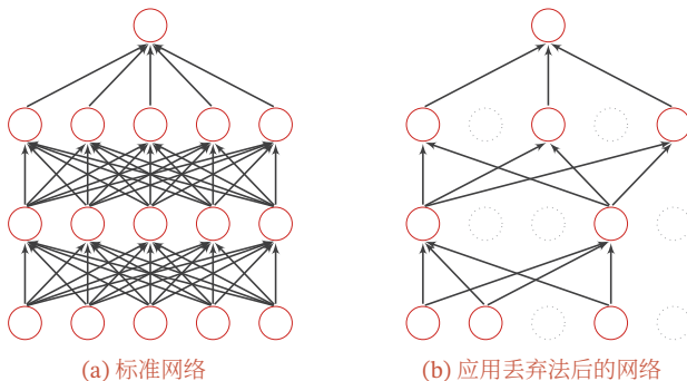
图 7.12 丢弃法示例
