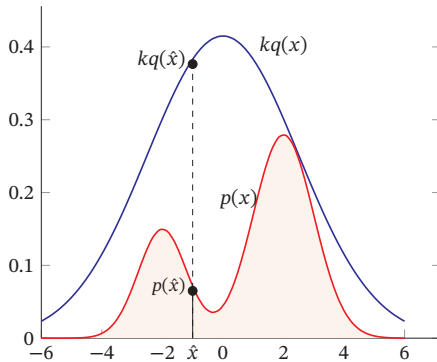
图 11.15 拒绝采样
