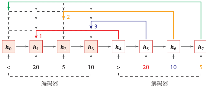
图 8.2 指针网络
