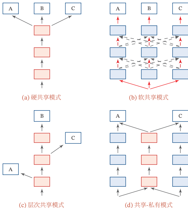
图 10.1 多任务学习中四种常见的共享模式
